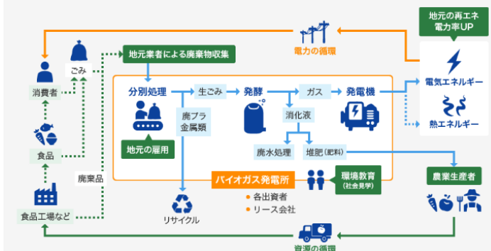
羽村バイオガス発電所が行う「食品廃棄物リサイクルのフロー」
